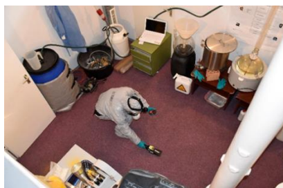
A felületiszennyezettség-mérő és dózisteljesítmény-mérő segítségével történő helyszíni felderítés
